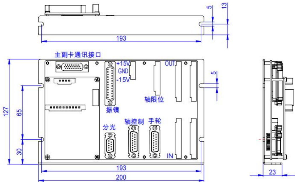
PCIE 端子板
