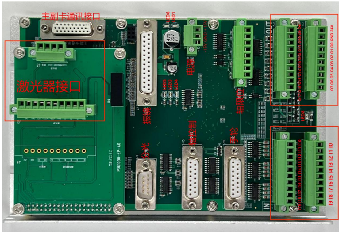
PCIE 端子板
